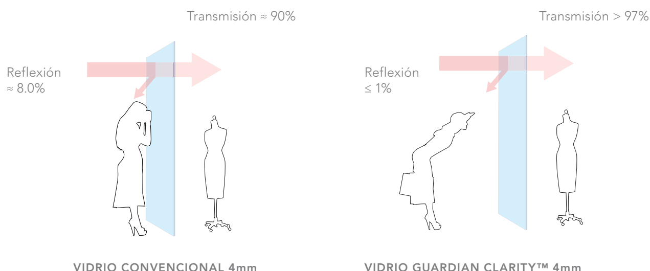
Comparativa prestaciones vidrio convencional vs Guardian Clarity™
