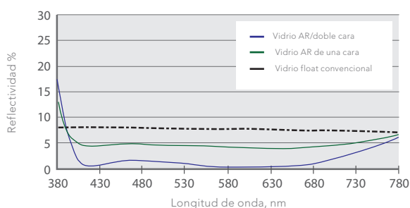
Reflectancia vs longitud de onda: Rvis típica < 0.4% por cara capa*
